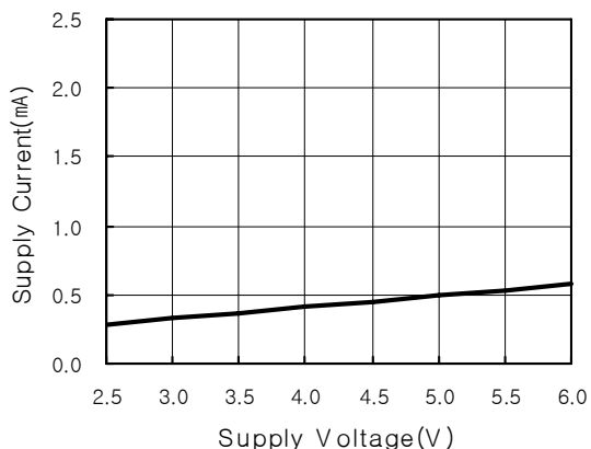
図.1 供給電圧と消費電流
