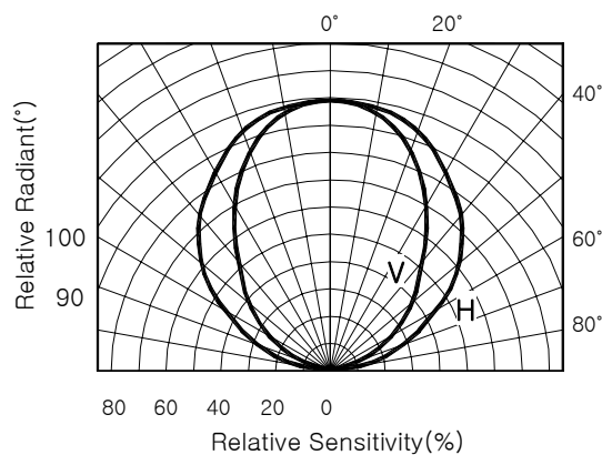
図.4 指向角
