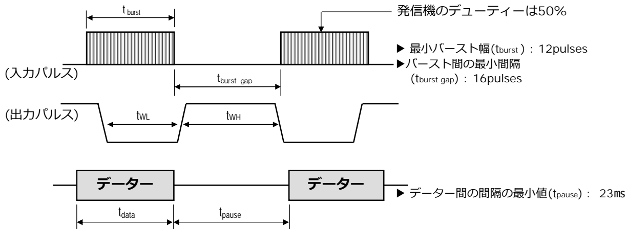
● 図1 .バースト波形、出力波形
